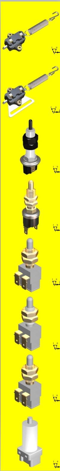
07 0102 TABLALI YAYLI FREN ŞALTERİ
